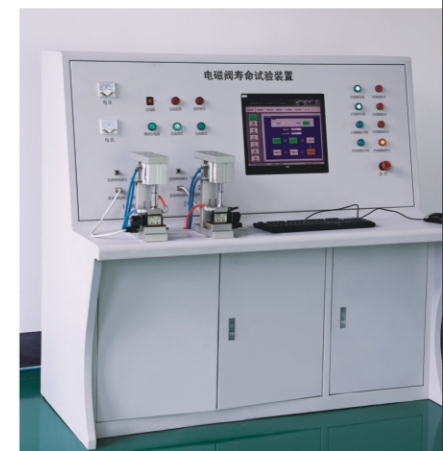
◎ 测试台 Test Board
